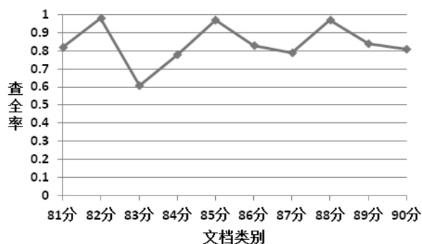
图 5 查全率
