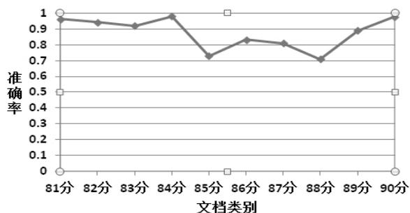
图 4 查准率
