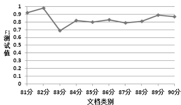
图 6 F 1 值
